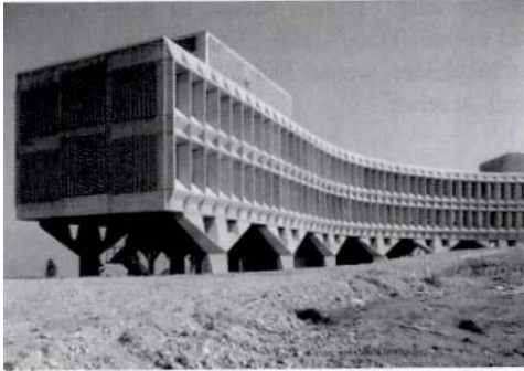
IBM-Forschungszentrum bei Nizza: Der gesamte Baukörper ruht auf sich dreifach gabelnden Betonstützen
